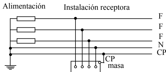
Esquema TN-S
