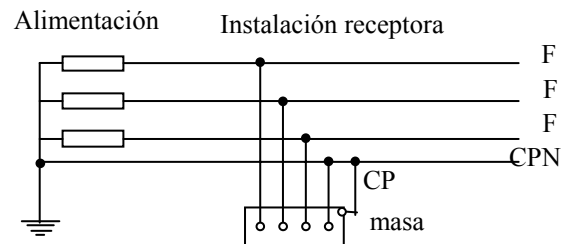
Esquema TN-C
