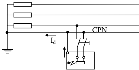
Esquema TN-C
