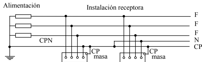
Esquema TN-C-S
