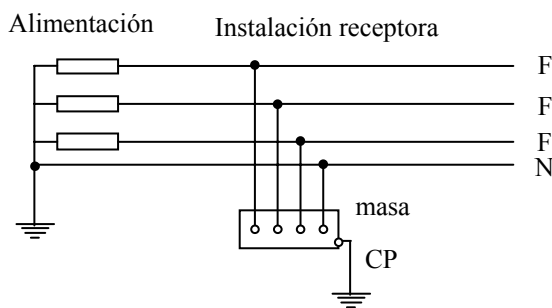
Esquema TT
