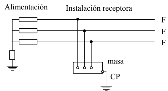
Esquema IT
